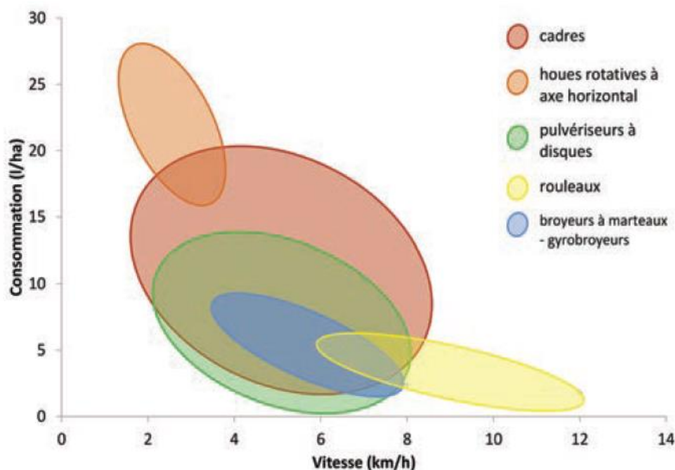
Figure 2 : Gamme de variation de consommation des différents outils inter-rang, en fonction de la vitesse de travail (Constant et al. , 2019)
